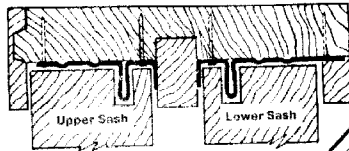
Jamb Section
